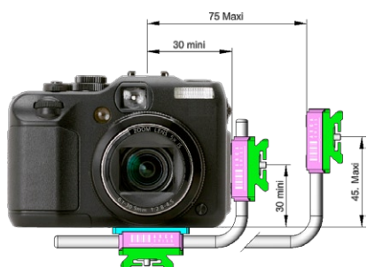
802304 mini L-Bracket
