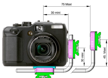
802304 mini L-Bracket
